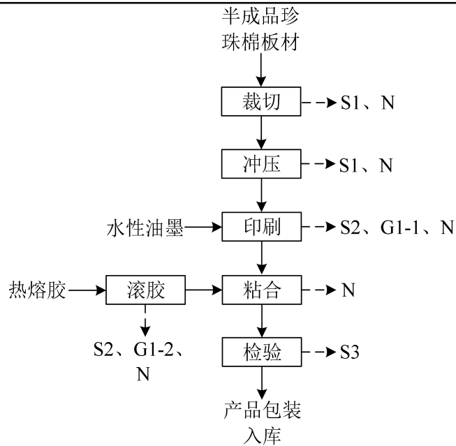
图2-1 珍珠棉生产工艺流程及产污环节图
