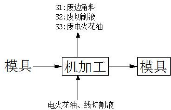
图 5-2 模具维修流程及产污环节图
