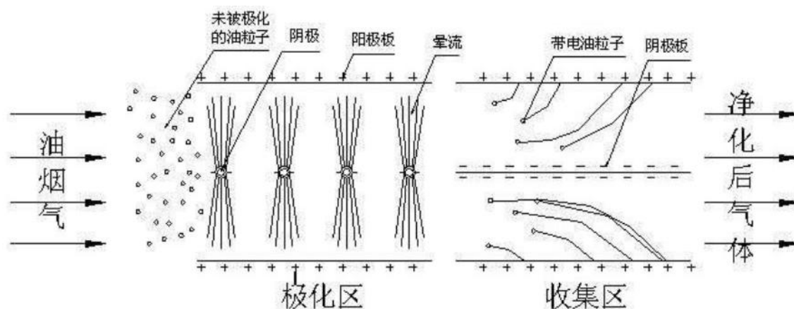
图 7-2 油烟净化器处理原理图
