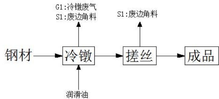
图 5-1 生产工艺流程及产污环节图
