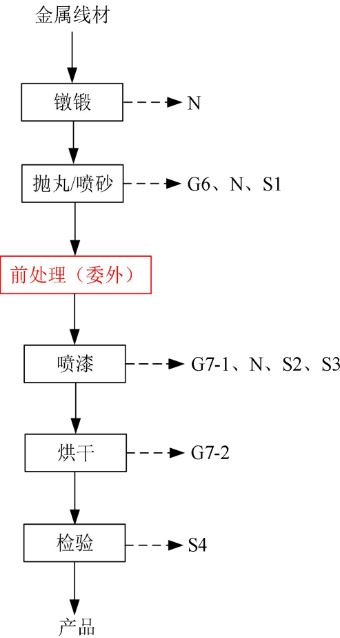
图5-3 紧固件生产工艺流程及产污环节
