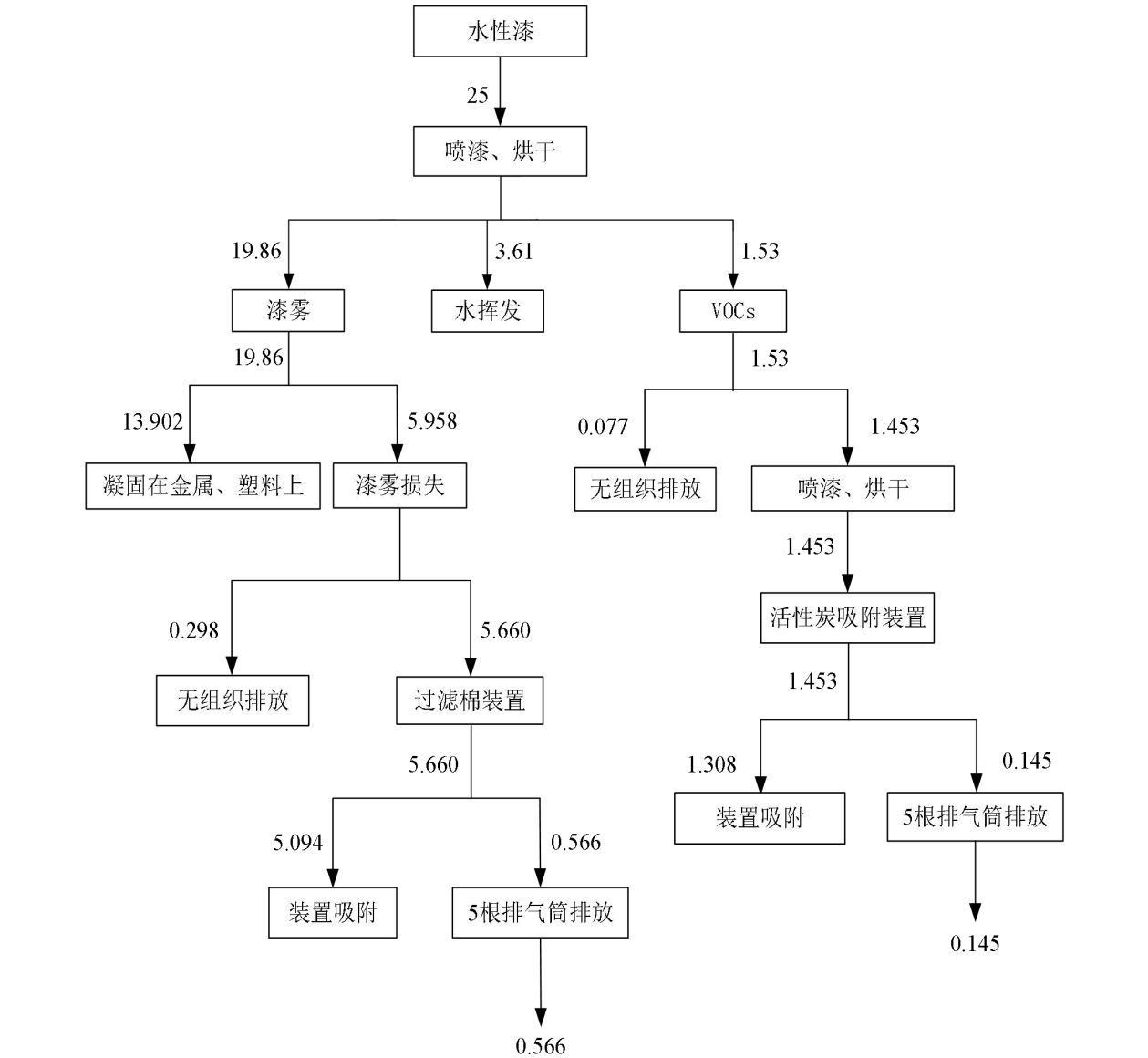
图 5-4 本项目水性漆物料平衡图 (t/a)
