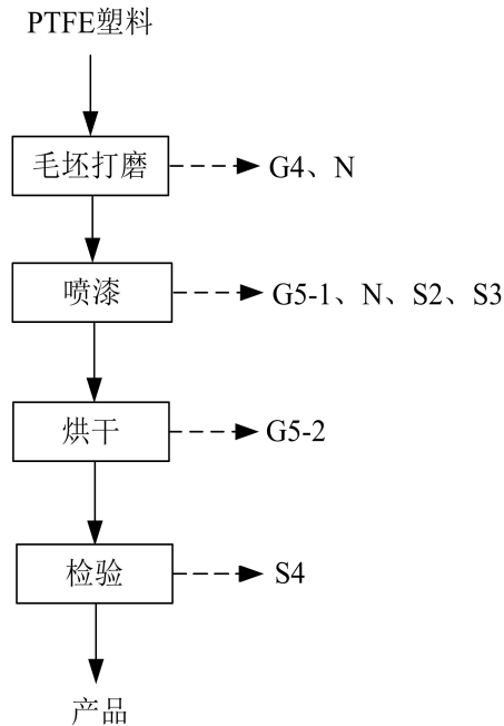
图5-2 汽车塑料配件生产工艺流程及产污环节
