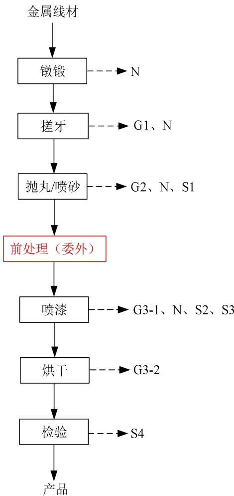
图 5-1 汽车金属配件生产工艺流程及产污环节图
