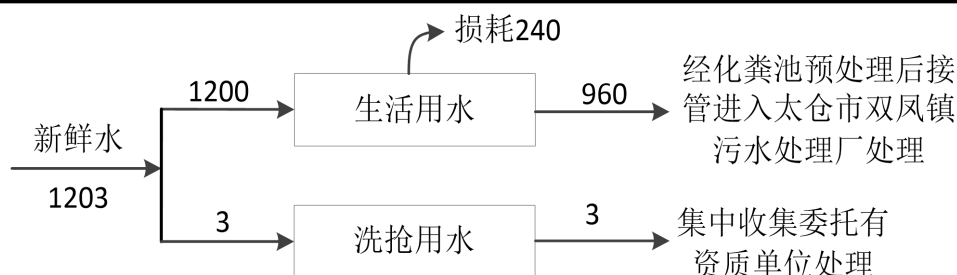
图 5-5 本项目水平衡图 (t/a)
