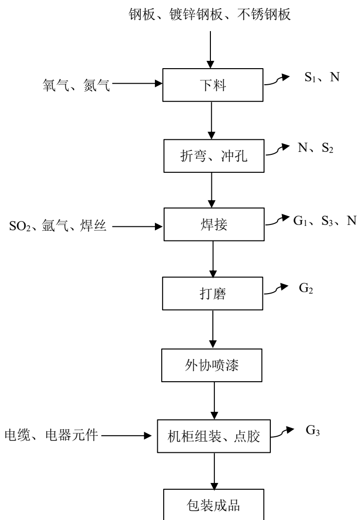
图 5-1 电气控制柜生产工艺及产污环节图
