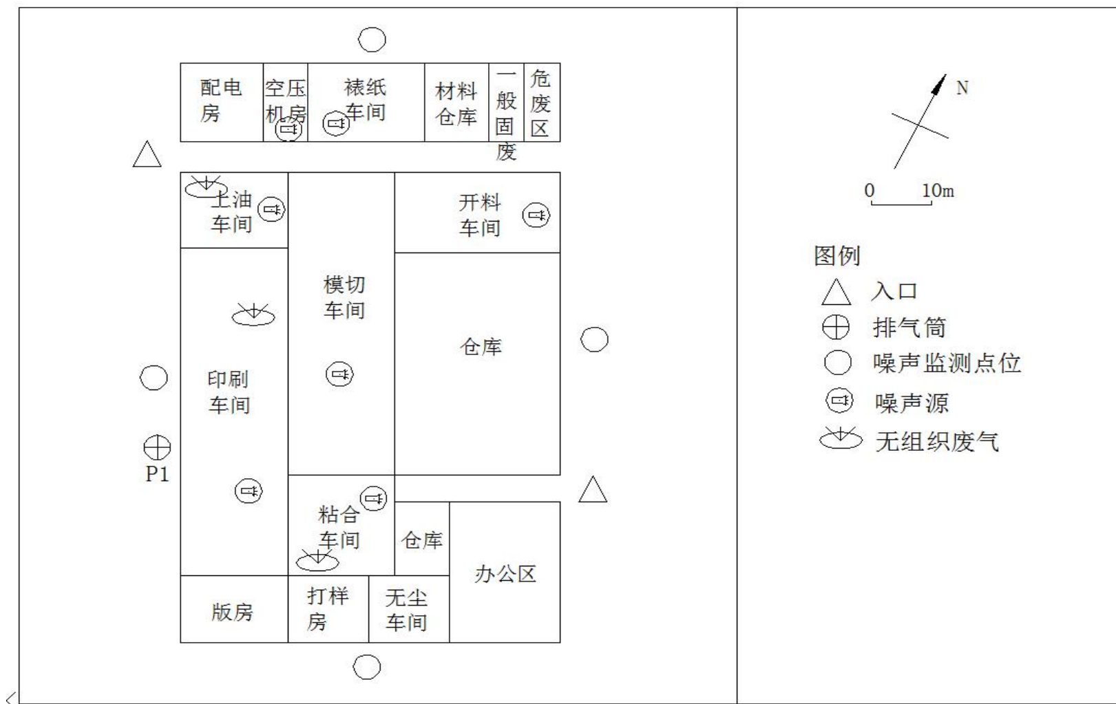
附图三 建设项目厂区平面布置图
