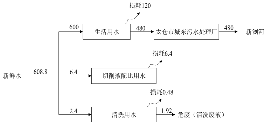
图 2-1 生产工艺流程图
