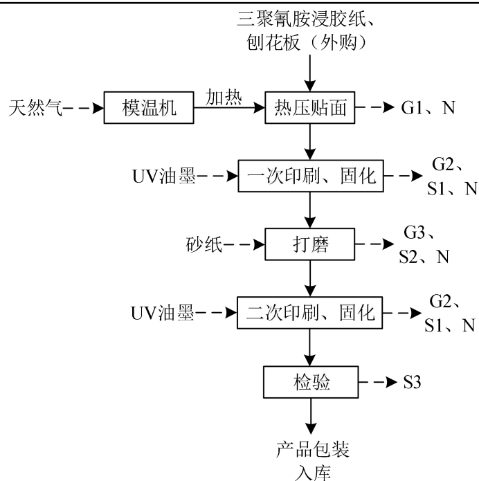
图 2-1 生态饰面板生产工艺流程及产污环节图
