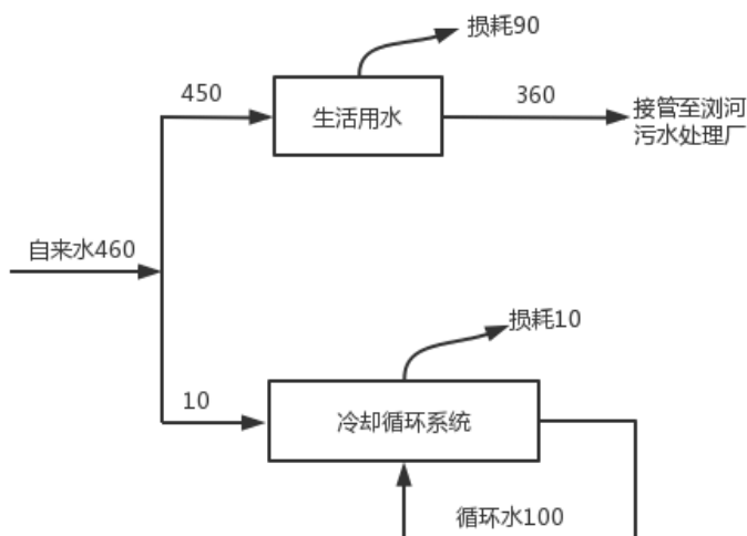
图 4-1 建设项目水平衡图 单位: t/a
