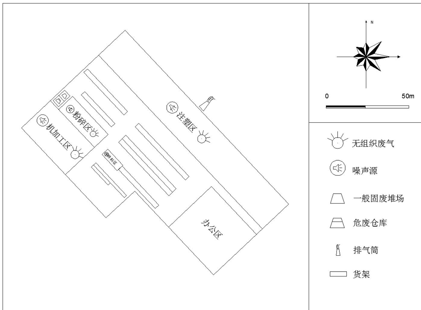
附图 3-1 本项目车间平面图
