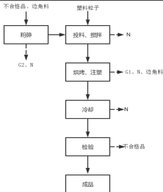
图 2-1 塑料制品生产工艺流程及产污环节图
