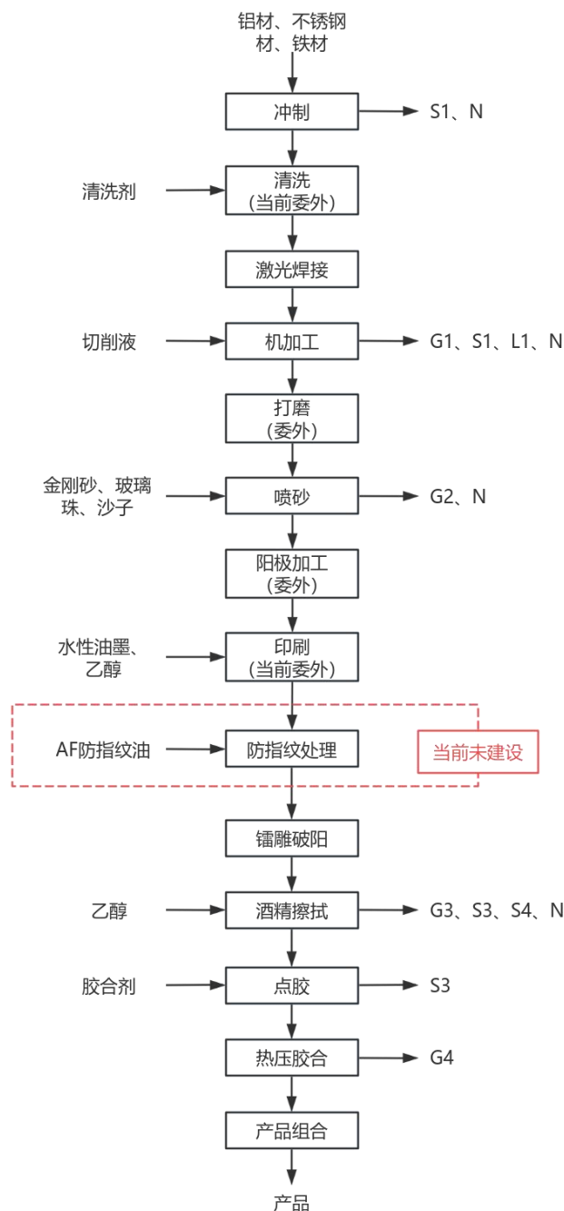
图 2-6 现有项目电脑配件、手机配件、医疗配件生产工艺流程和产污环节图
