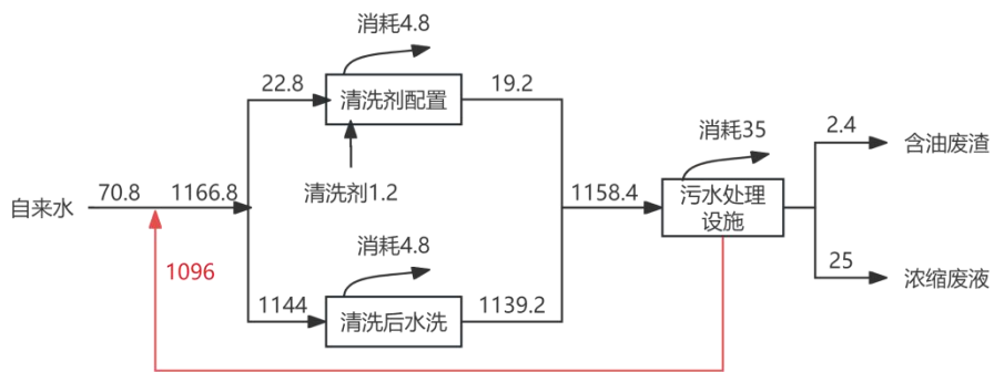
图 2-1 本次扩建项目水平衡图 (t/a)
