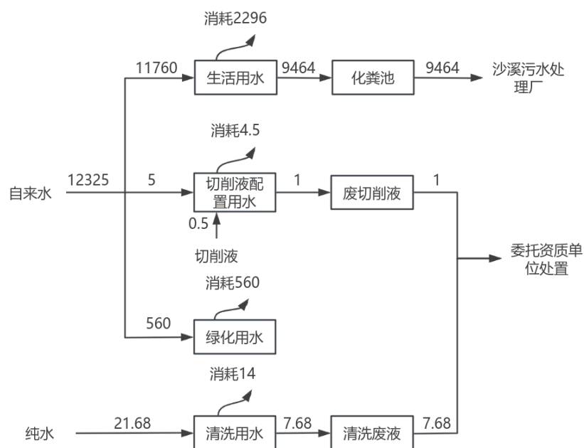
图 2-7 现有项目水平衡图
