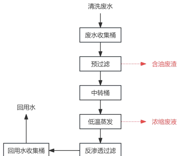
图 4-1 生产废水处理工艺流程图
