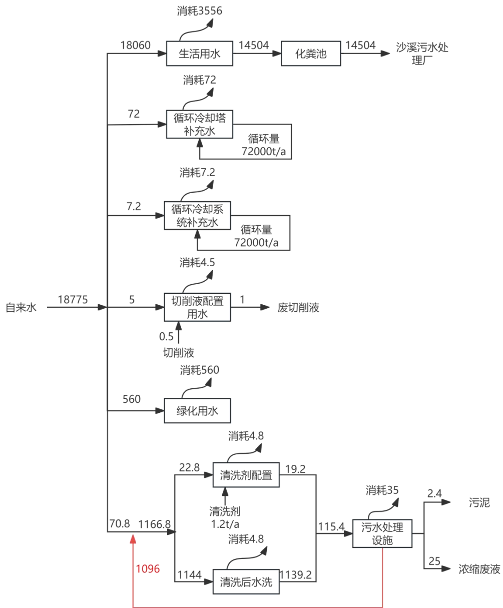
图 2-2 全厂水平衡图 (t/a)
