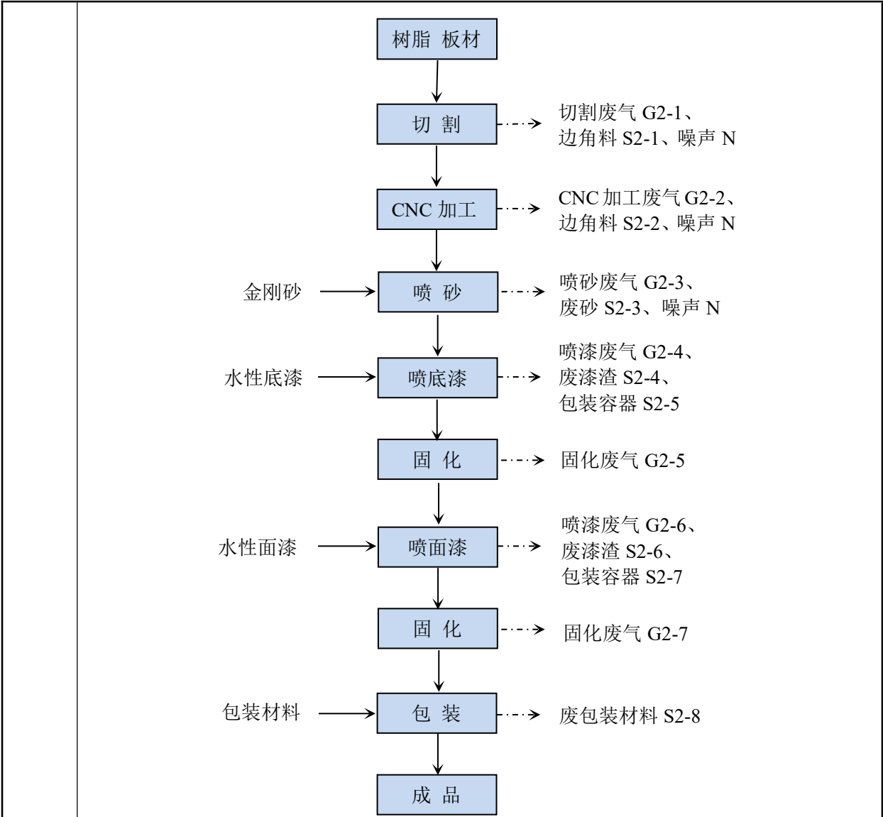
图 2-3 树脂模具生产工艺流程及产污环节图
