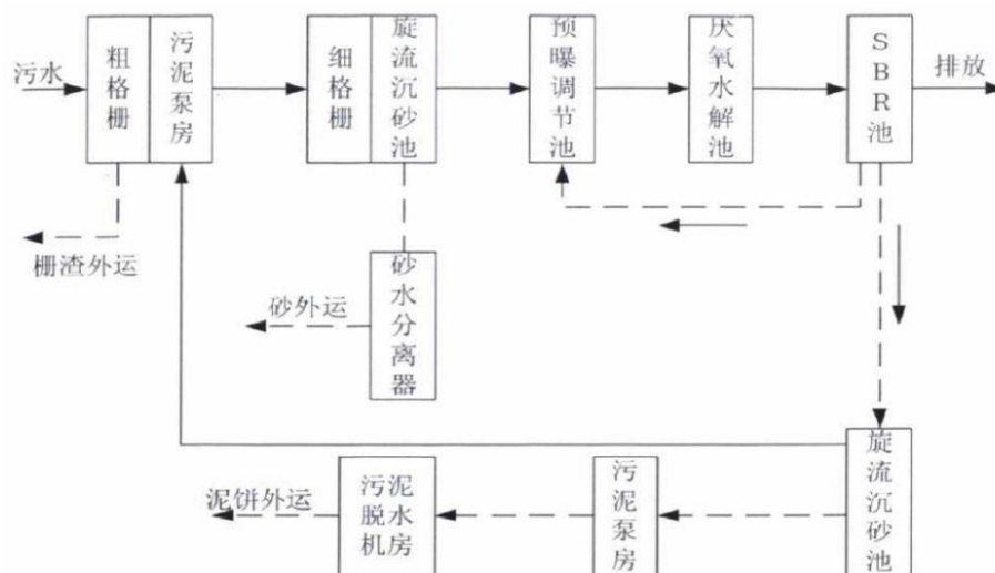
图 4-3 太仓市沙溪污水处理厂污水处理工艺流程图
