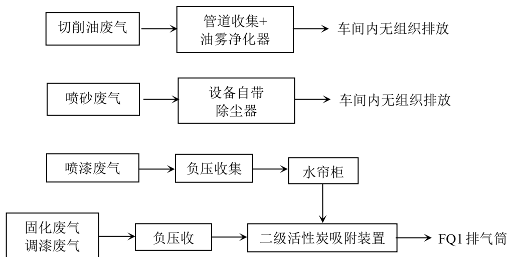
图4-2 本项目废气处理工艺流程图
