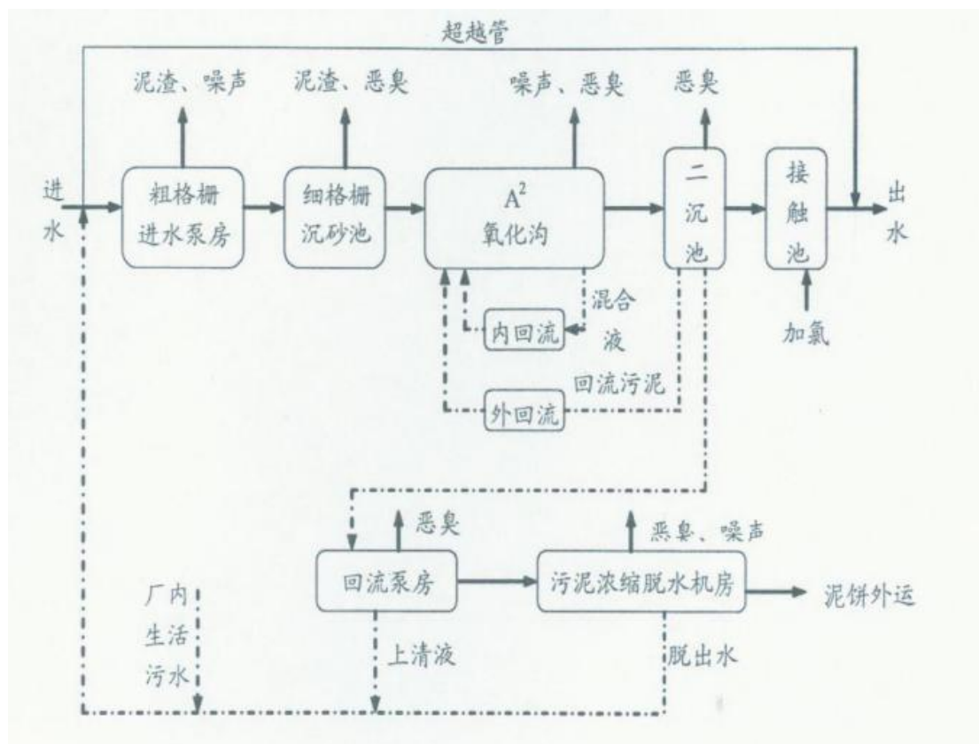
图 2.1-1 环评中生产工艺及产污节点图
