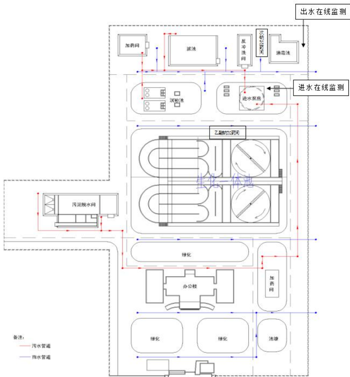
图 3-2 车间平面布置图
