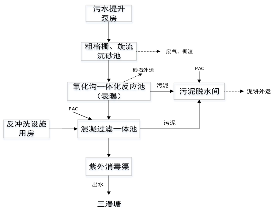
图 3-3 生产工艺及产污节点图
