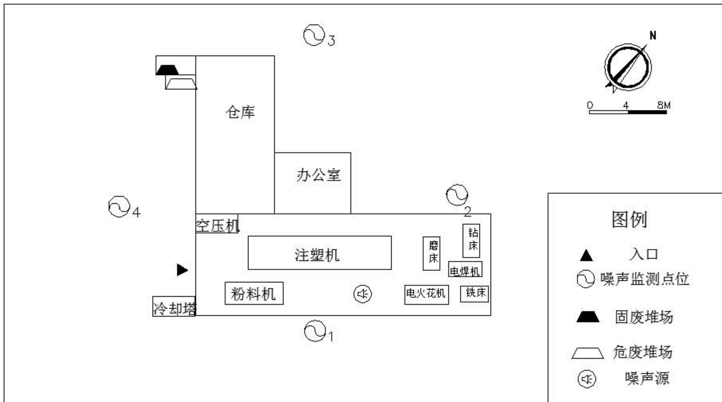
附图三 建设项目平面布置图
