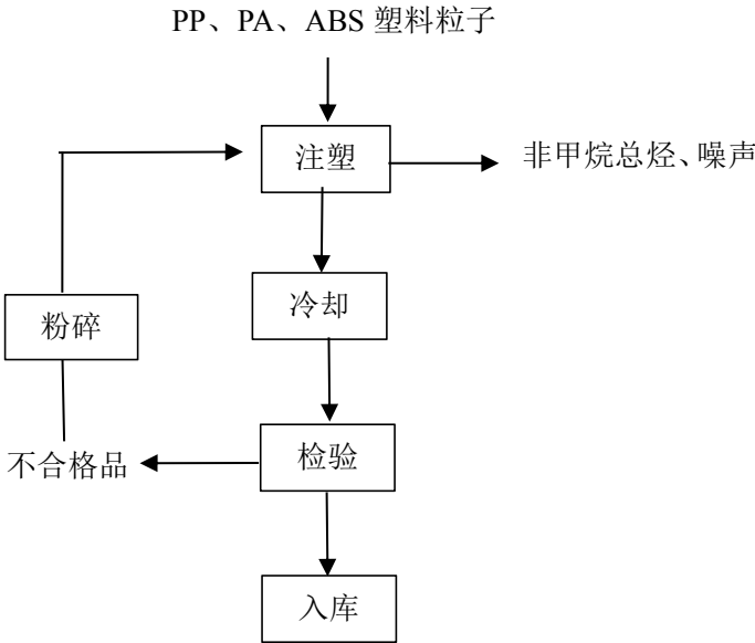
图 1 塑料制品生产工艺流程图
