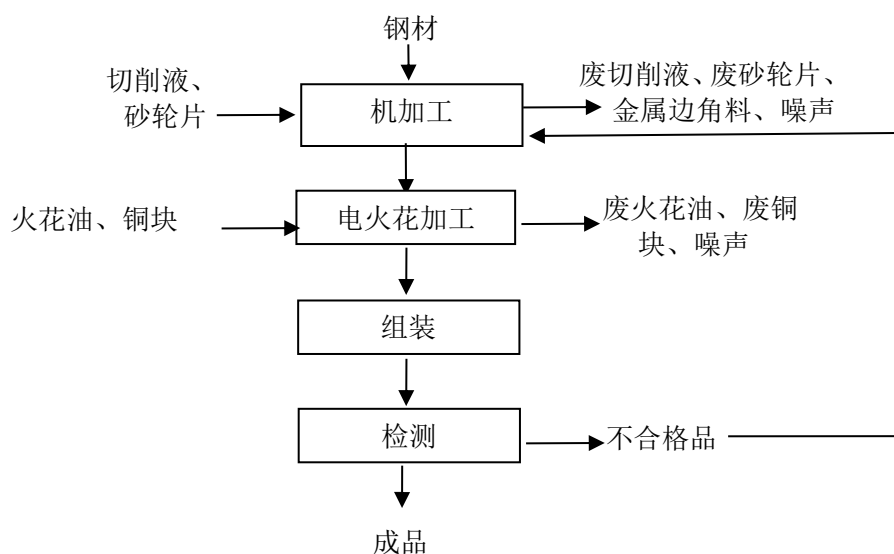
图 2 模具生产工艺流程图
