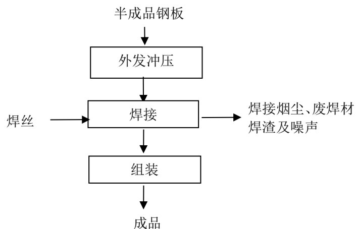
图3 金属制品生产工艺流程图
