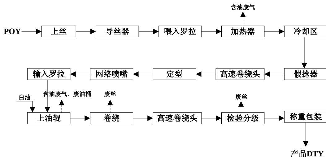
图 1-1 加弹丝生产工艺流程及产污环节图
