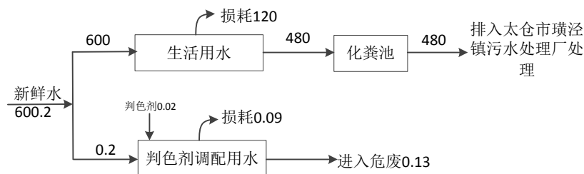
图 5-3 扩建后全厂水平衡图 (t/a)
