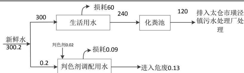
图 5-2 扩建项目水平衡图 (t/a)
