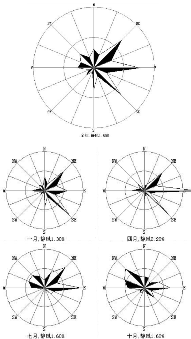
图 2-1 太仓市风玫瑰图
