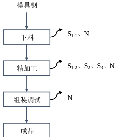
图5-1 冲压模具工艺流程及产污环节图
