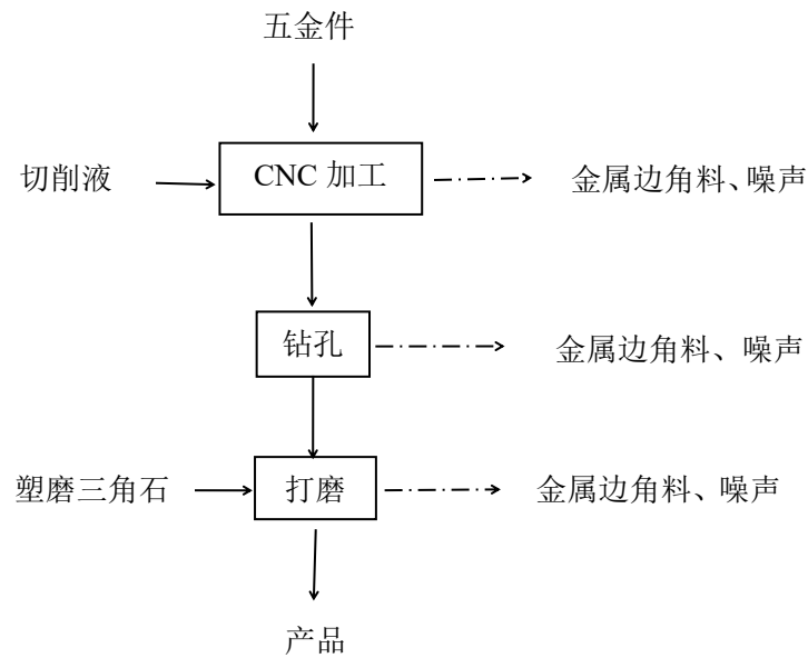
图 3 建设项目金属件生产工艺流程图
