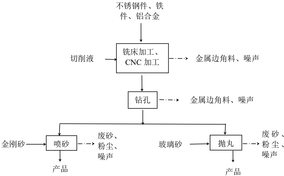
图2 建设项目自动化零部件生产工艺流程图
