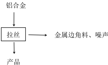
图 3 建设项目矩形零部件生产工艺流程图
