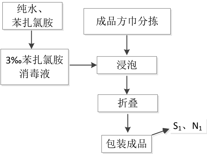
图 5-1 湿巾生产工艺流程图
