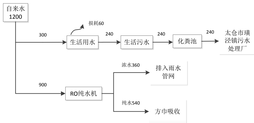
图 5-3 本项目水平衡图 （单位：t/a）
