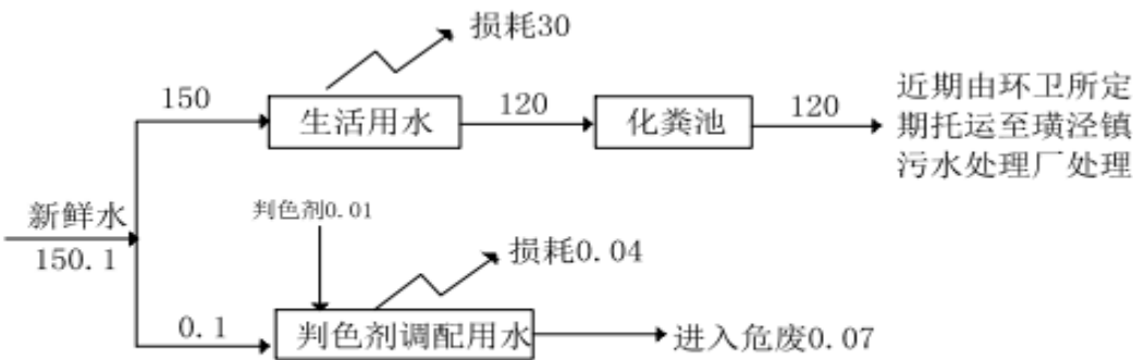
图 1-2 原有项目水平衡图 (t/a)
