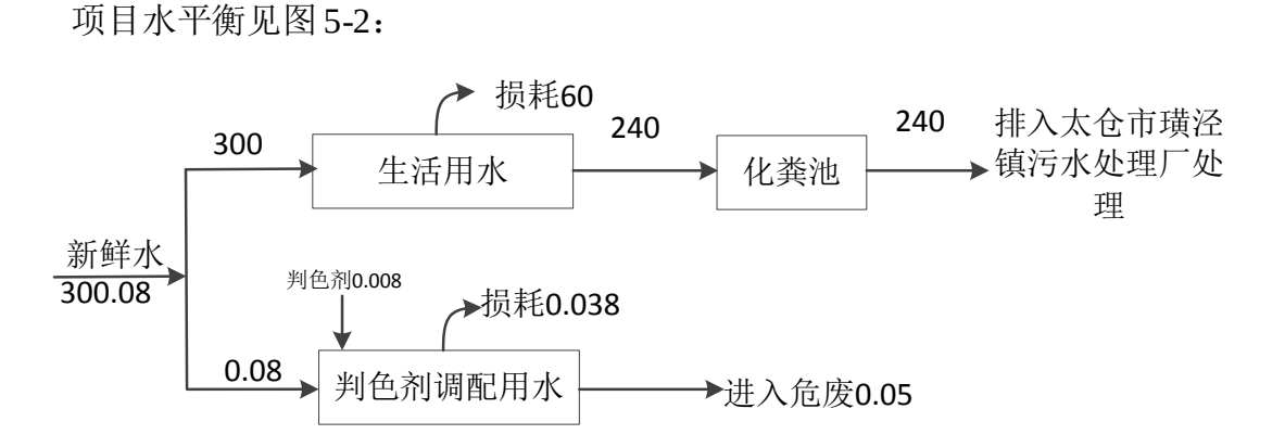
图 5-2 扩建项目水平衡图（t/a）
