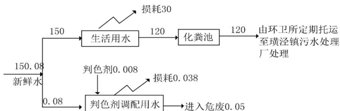
图 1-2 原有项目水平衡图 (t/a)
