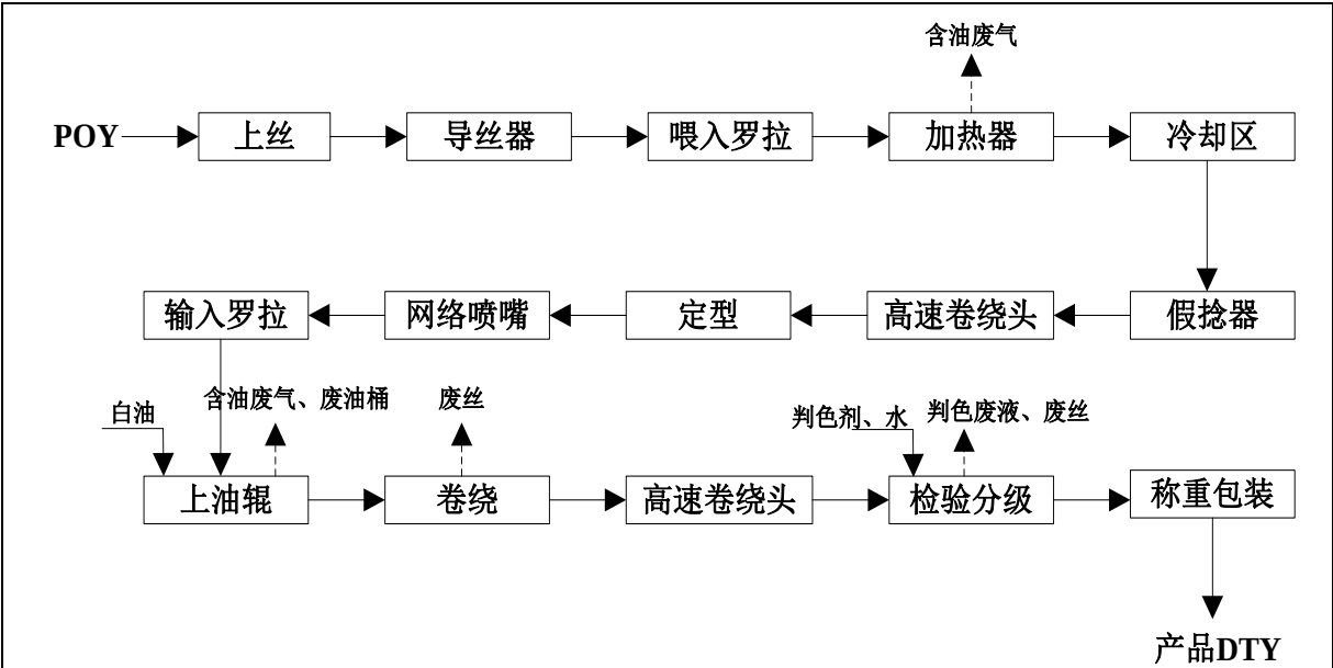
图 1-1 加弹丝生产工艺流程及产污环节图
