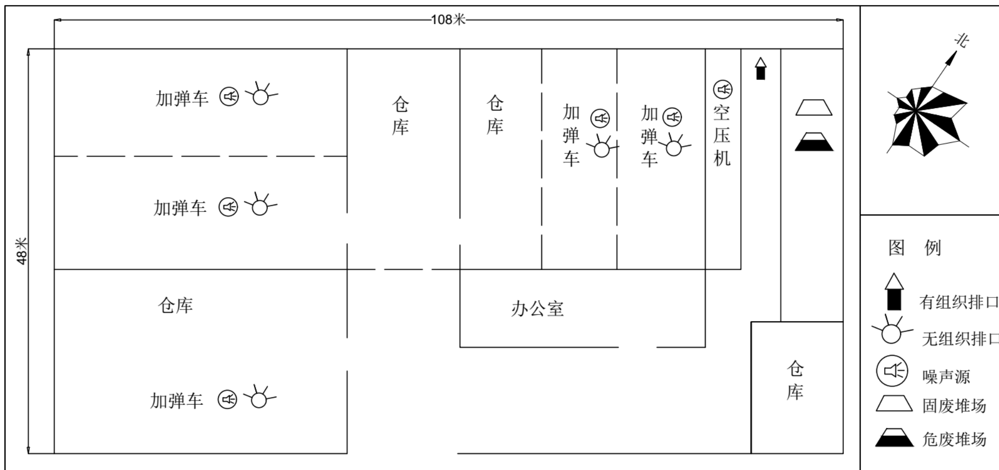
附图 3 厂区平面布置图
