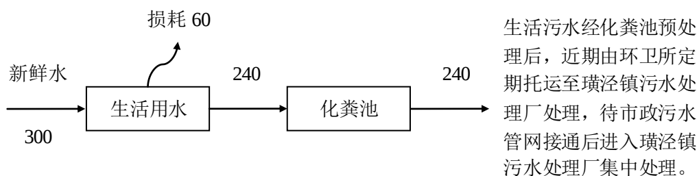
图 5-2 扩建项目水平衡图 (t/a)
