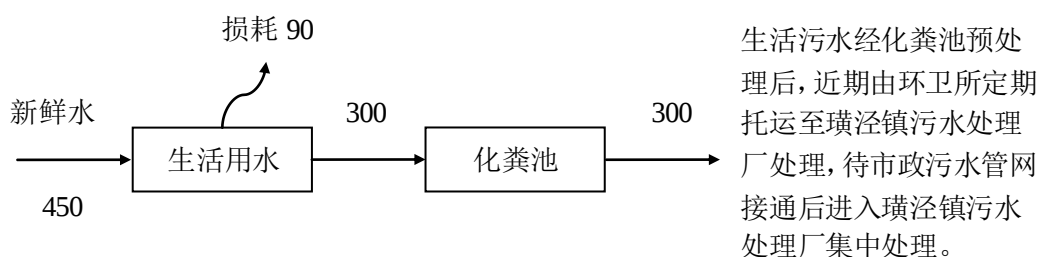
图 5-2 扩建项目水平衡图 (t/a)
