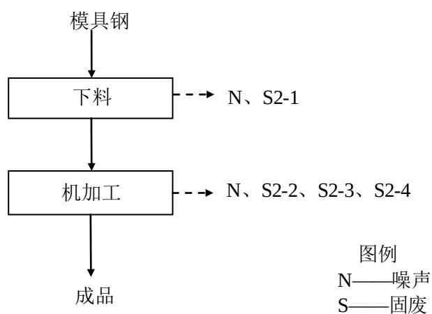
图 5-2 模具生产工艺流程图
