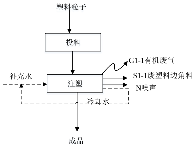
图 5-1 塑料制品生产工艺流程图
