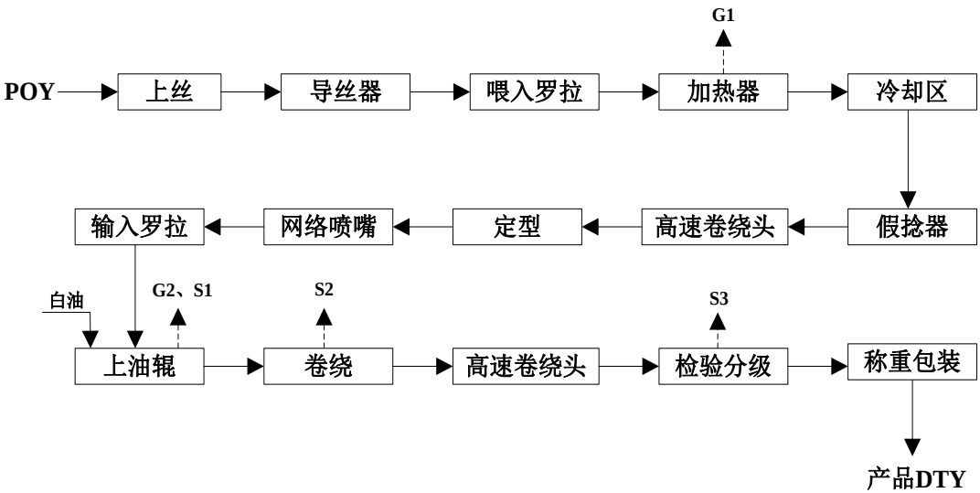
图 5-2 涤纶 DTY 加弹丝生产工艺流程及产污节点图
