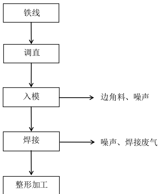
图 1-1 五金制品生产工艺流程图
