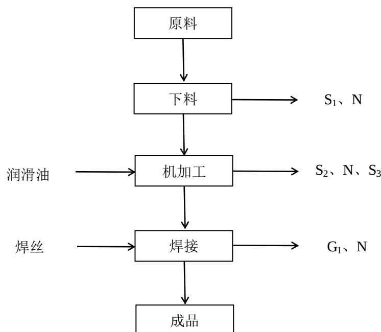
图 5-1 搬迁项目生产工艺及产污环节图
