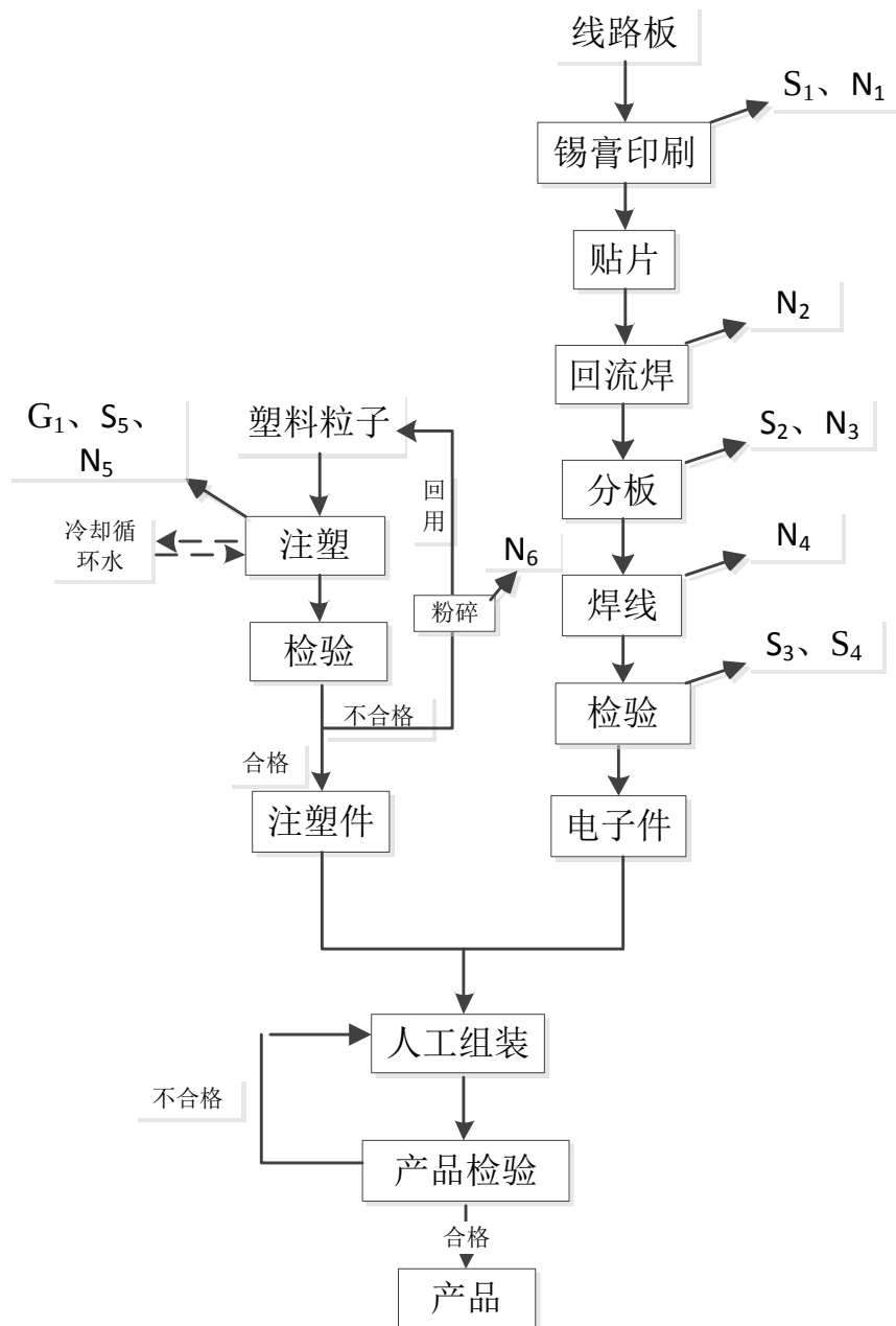
图 5-1 建设项目生产工艺流程图
