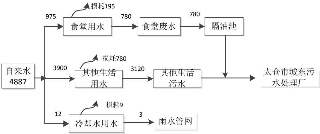
图 5-3 水平衡图 （单位：t/a）
