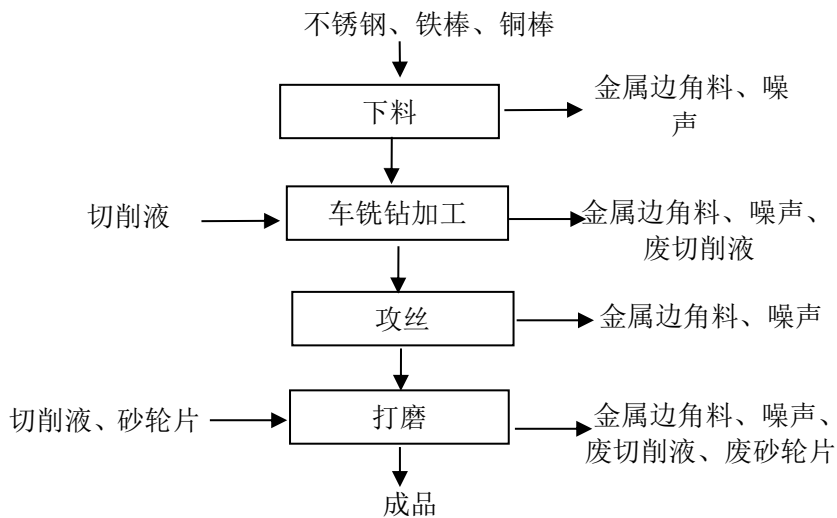
图 1 五金产品生产工艺流程图
