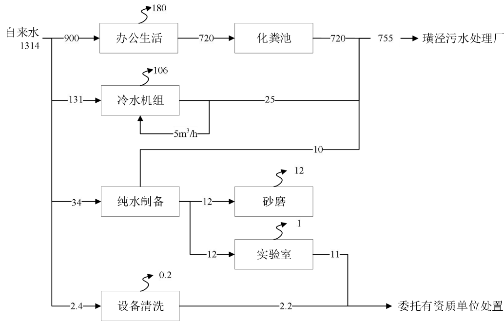
图2-3 本项目水平衡图 (t/a)
