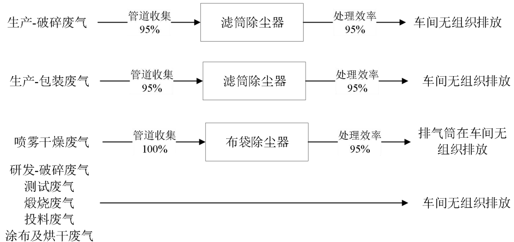
图4-1 本项目废气处理方式示意图
