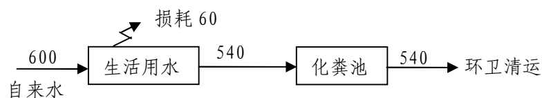
图1 建设项目用排水平衡图 (单位 t/a)
