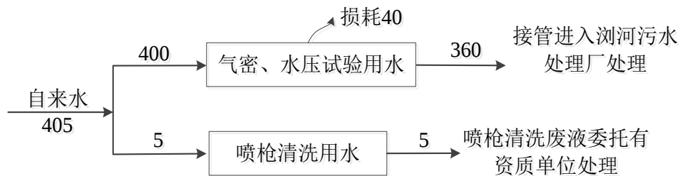
图 5-3 本项目水平衡图 单位: t/a
