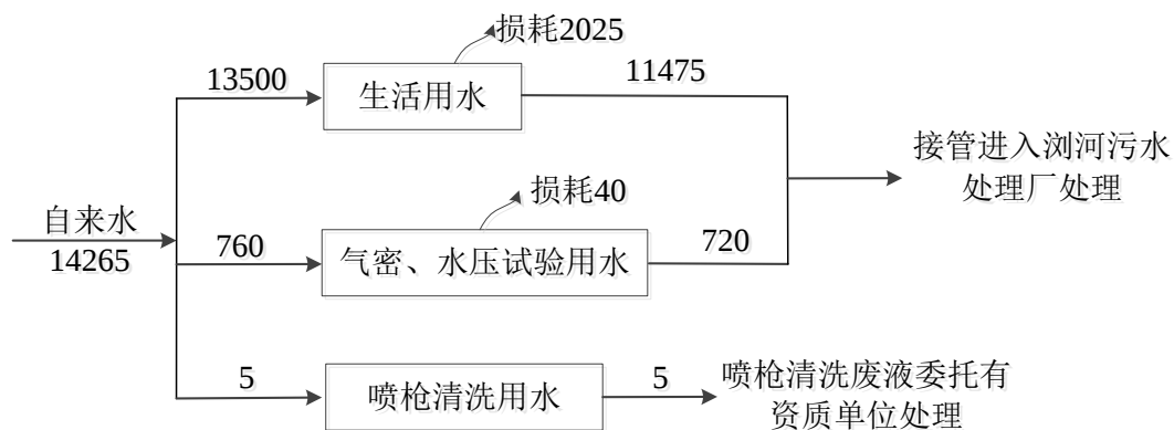
图 5-4 全厂水平衡图 单位: t/a
