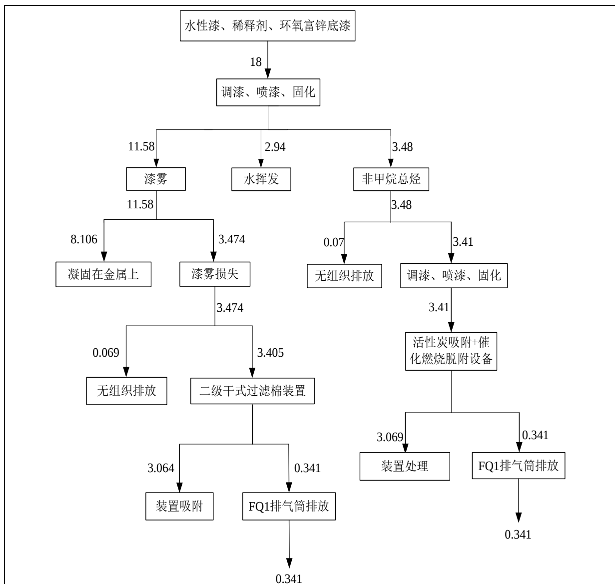
图 5-5 本项目水性漆物料平衡图 (t/a)
