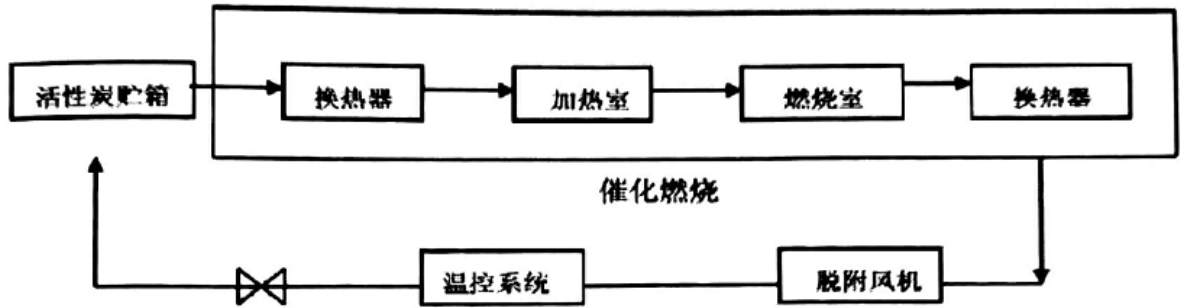
图 7-1 活性炭吸附+催化燃烧脱附设备
