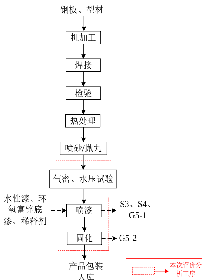
图 5-2 现有项目工艺流程及产污环节图
