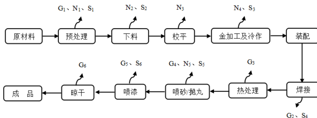
图 1-2 生产工艺流程及产污环节图
