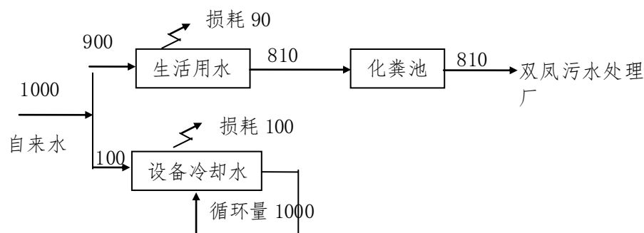
图2 建设项目用排水平衡图 (单位 t/a)
