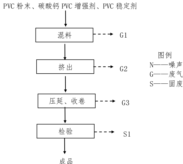
图 1 PVC 片卷材生产工艺流程图
