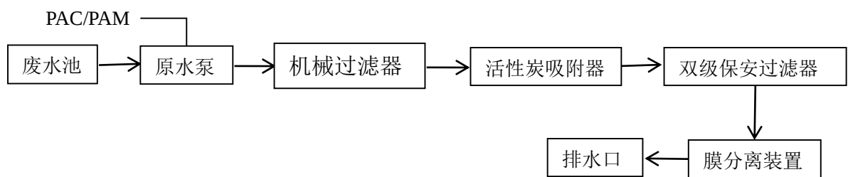
图 7-1 清洗废水处理工艺
