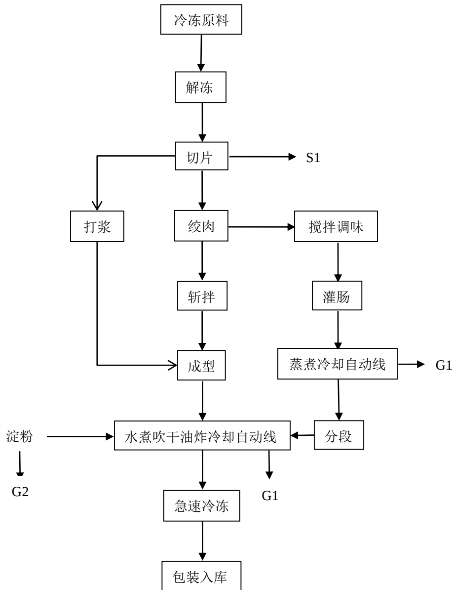
图 5-1 肉制品加工工艺及产污环节图
