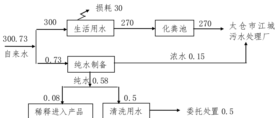
图 3 建设项目全厂用排水平衡图 (单位 t/a)
