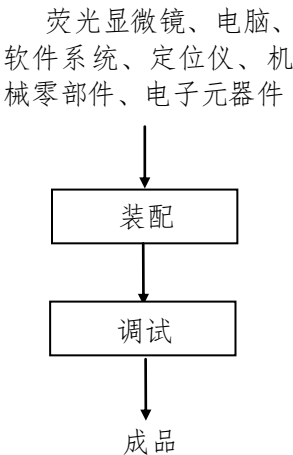
图 1 细胞样本分离仪生产工艺流程图
