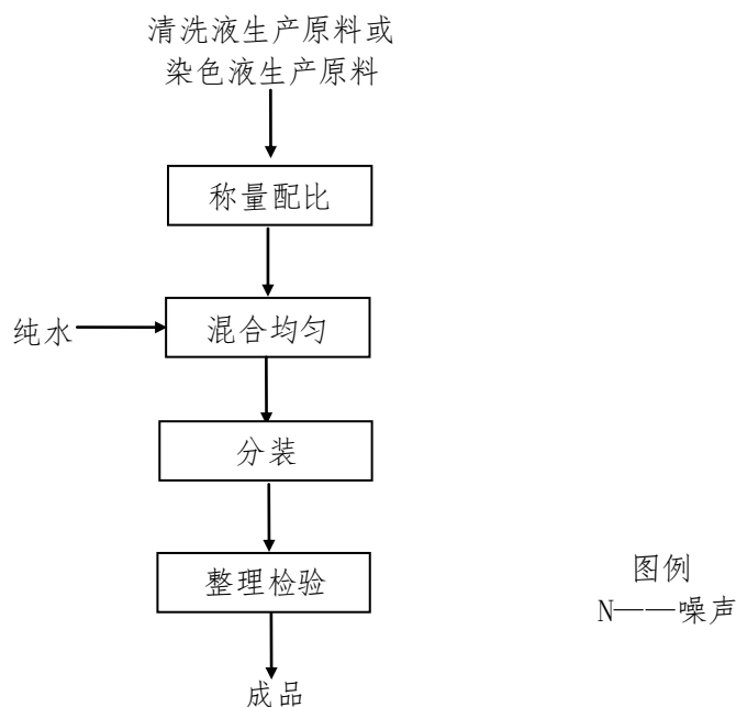
图2 细胞样本检测试剂生产工艺流程图
