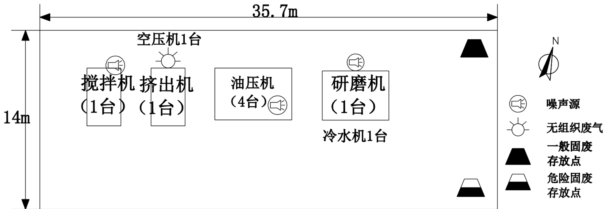
附图 3 项目生产车间平面布置图
