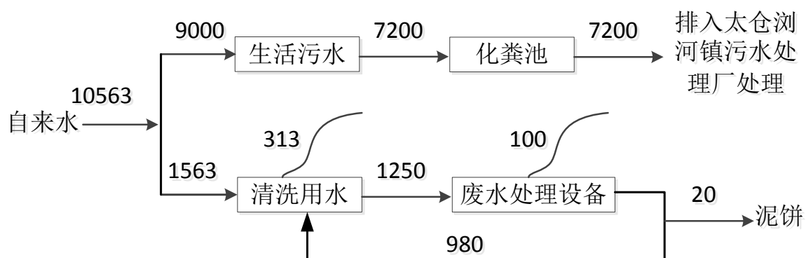
图 5-3 本项目水平衡图 (t/a)
