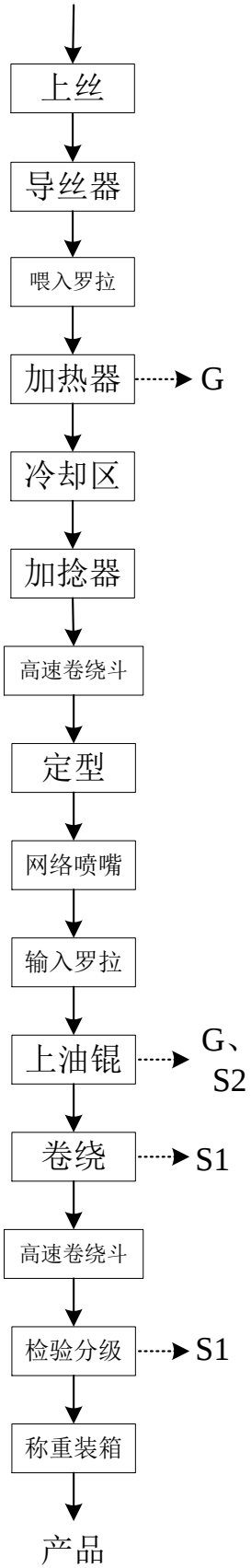
图 1-1 本项目生产工艺及产污环节图
