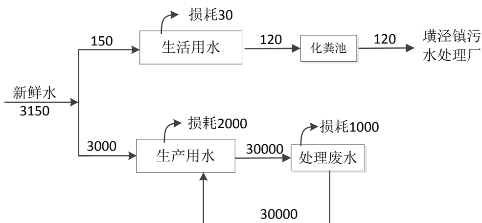
图 5-2 扩建项目水平衡图 单位： t/a
