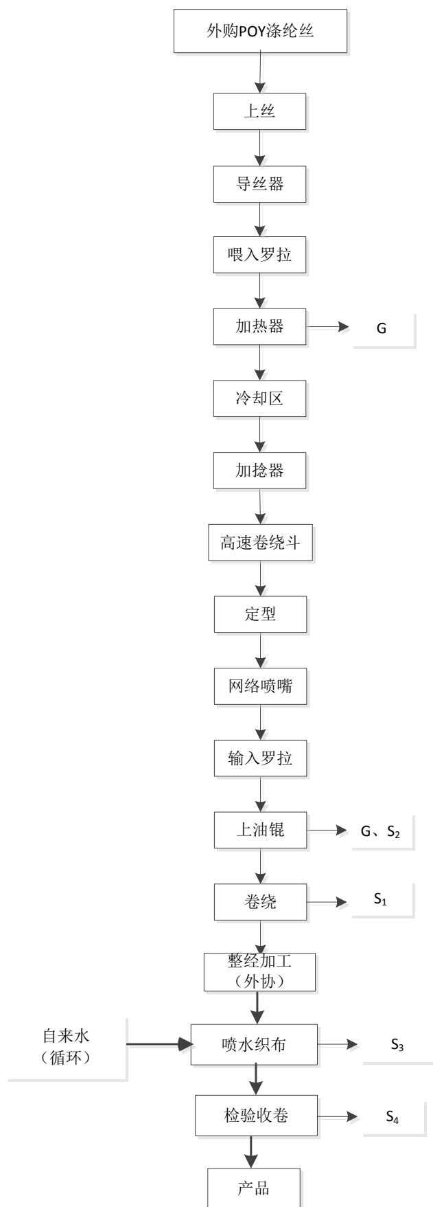
图 5-1 本项目生产工艺及产污环节图
