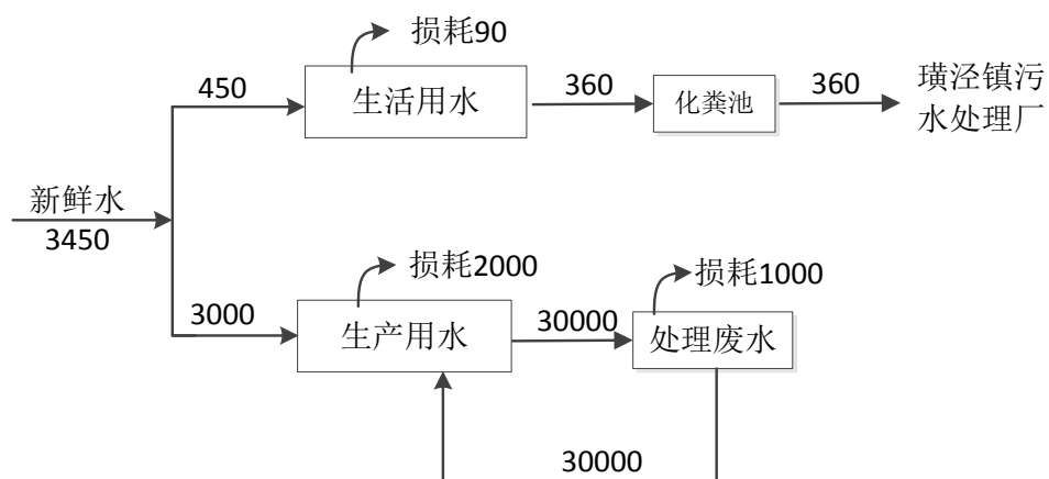
图 5-3 扩建后全厂水平衡图 单位： t/a
