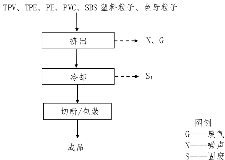
图 1 生产工艺流程图
