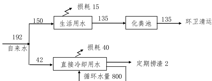
图 2 建设项目全厂用排水平衡图 (单位 t/a)
