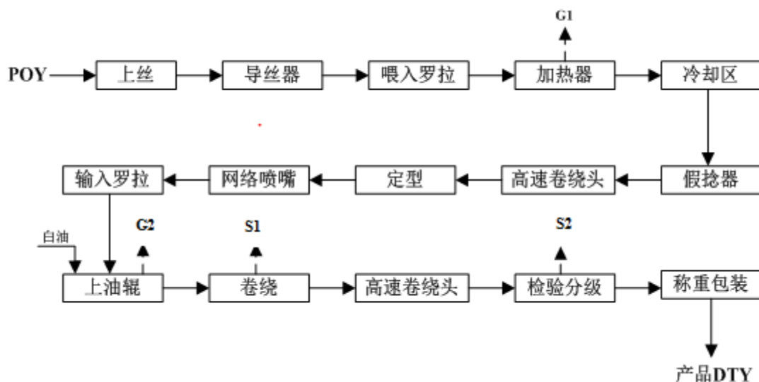
图 5-1 涤纶 DTY 加弹丝生产工艺流程及产污节点图
