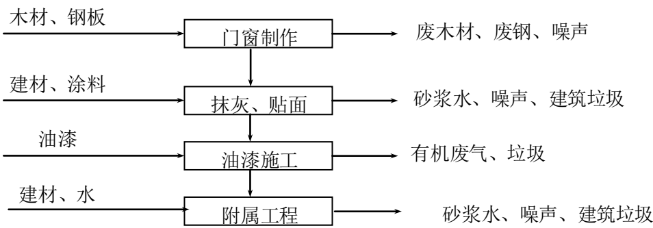
图 5-1 本项目施工期建筑工艺流程图
