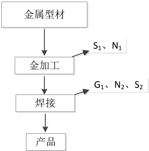
图 5-1 建设项目生产工艺流程图
