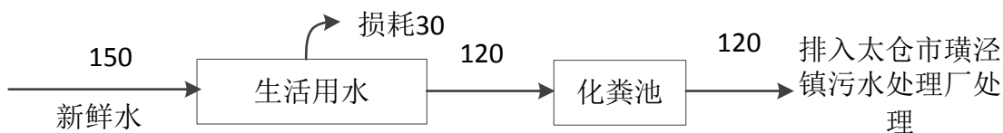
图 5-2 扩建项目水平衡图 (t/a)
