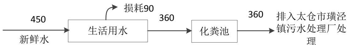
图 5-2 扩建项目水平衡图 (t/a)
