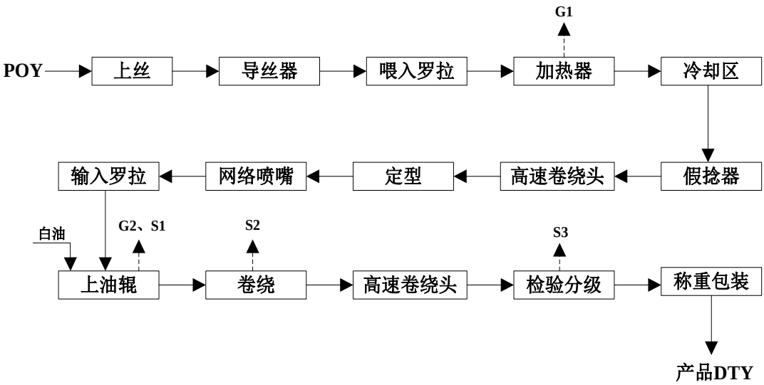
图 5-1 加弹丝生产工艺流程及产污节点图
