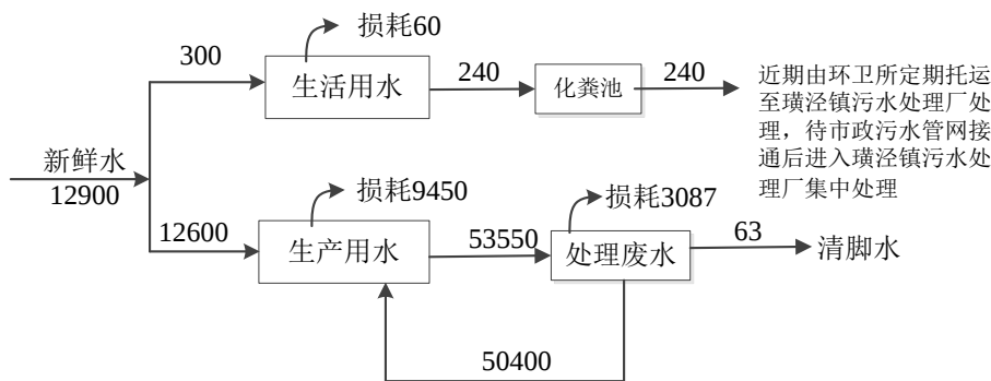
图 5-3 本项目水平衡图 (t/a)
