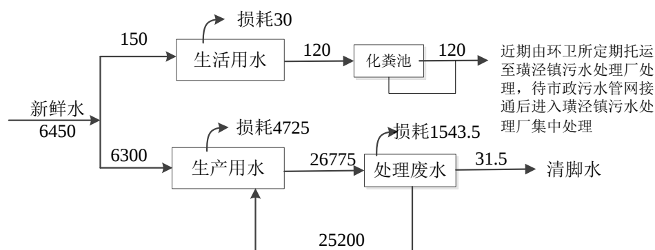
图 5-2 本项目水平衡图（t/a）
