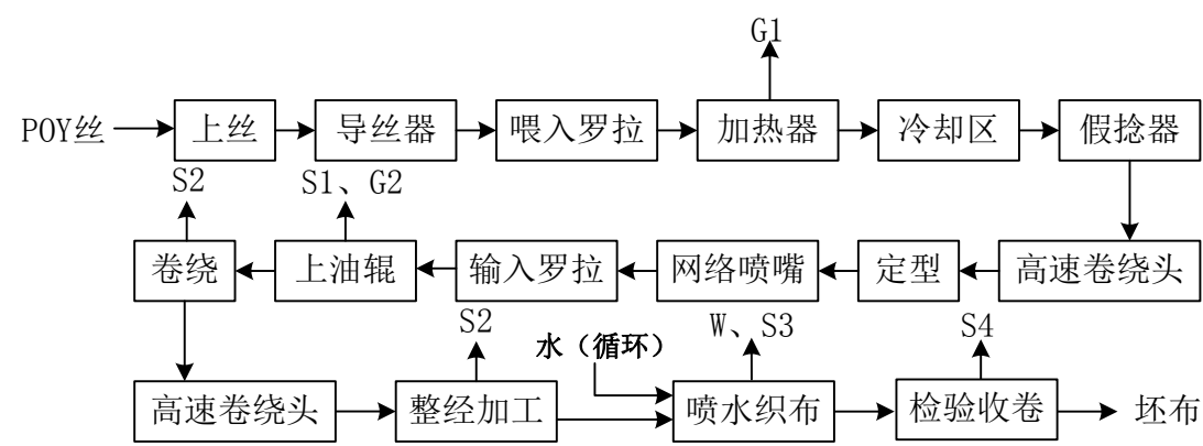
图 5-1 本项目生产工艺流程及产污节点图
