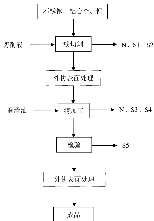
图 5-1 汽车零部件生产设备生产工艺及产污环节图
