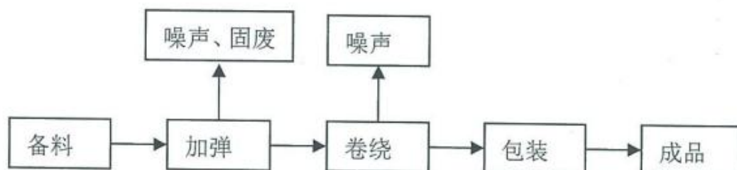
图 1-1 加弹丝生产工艺流程及产污环节图
