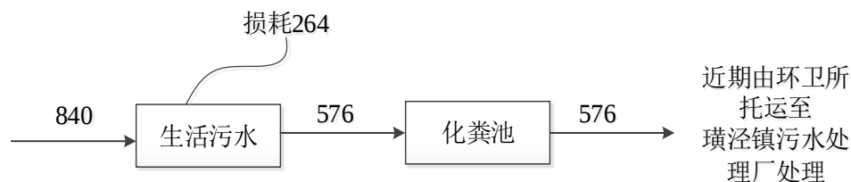
图 5-3 全厂水平衡图 (t/a)
