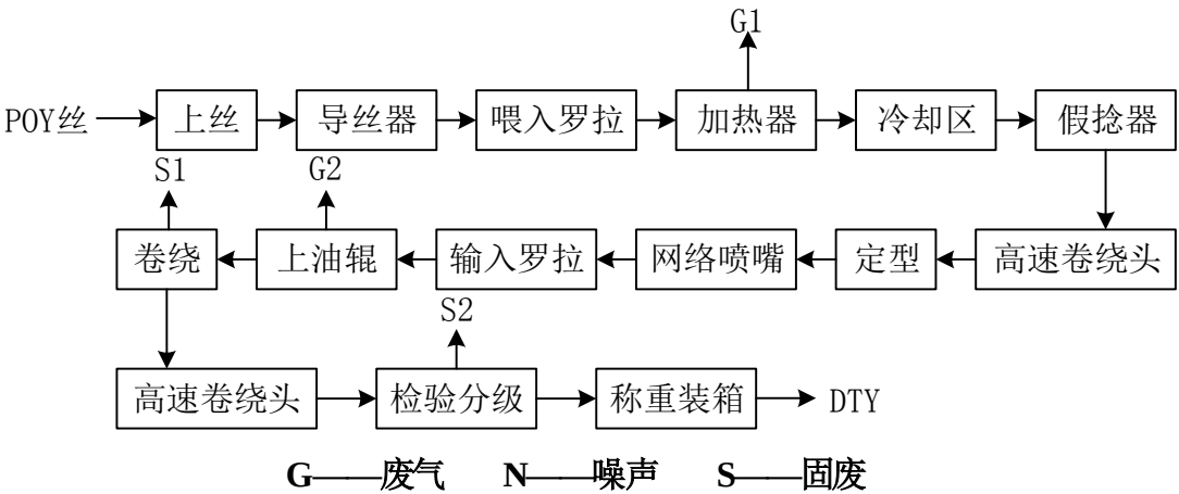
图 5-1 涤纶 DTY 加弹丝生产工艺流程及产污节点图
