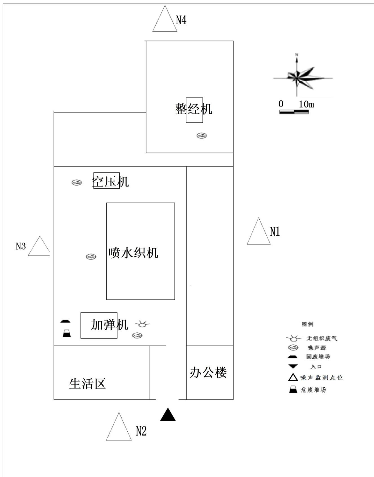
附图 3 项目平面布置图
