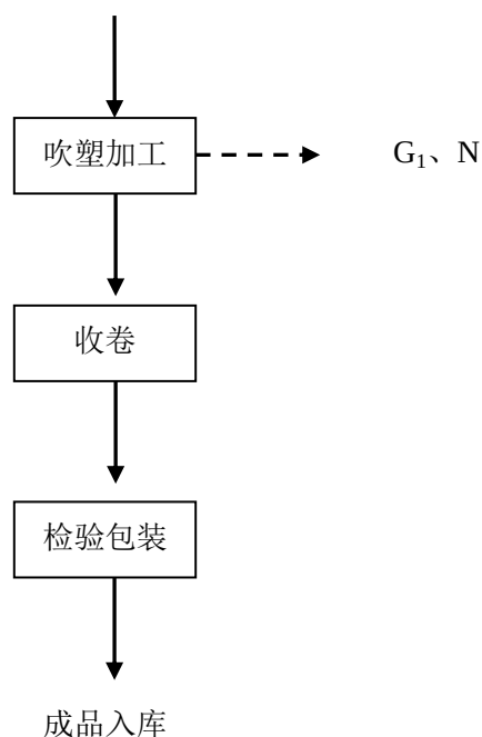
图 5-1 项目生产工艺及产污环节图
