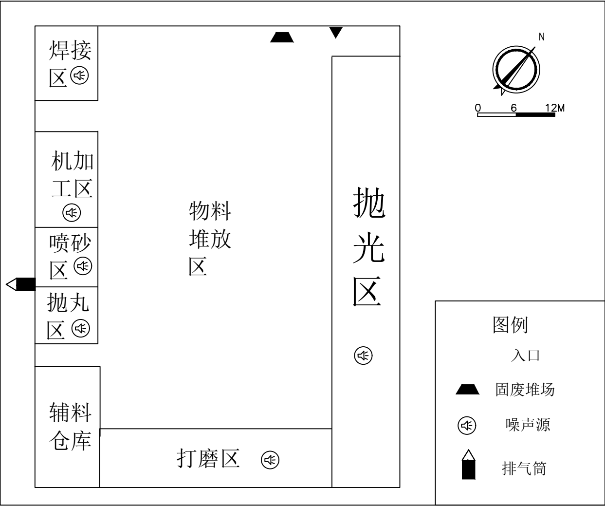
附图三 建设项目平面布置图
