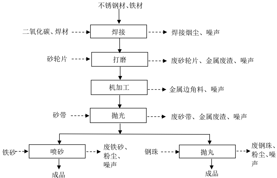
图 1 生产工艺流程图
