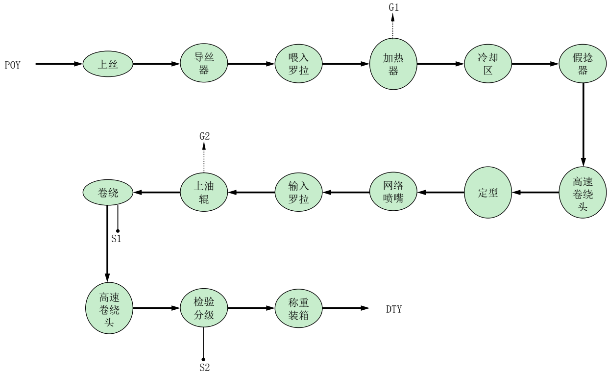
图 5-1 加弹丝生产工艺流程及产污环节图
