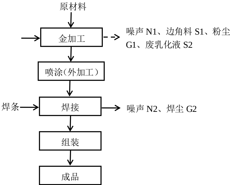
图 5-1 建设项目生产工艺流程图
