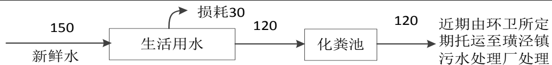
图 5-2 本项目水平衡图 (t/a)
